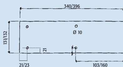
Platines de fixation (10/200 mm)
