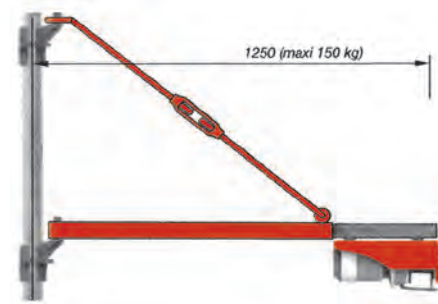
Potence portée de 1250 mm (poids : 150 kg)
