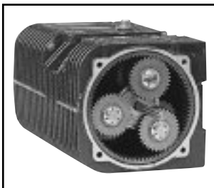
Réducteur planétaire.
